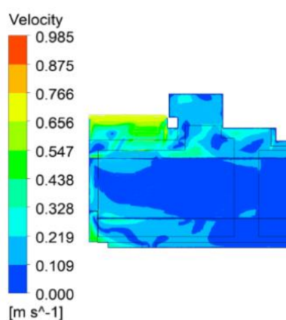
速度云图（改造后）
