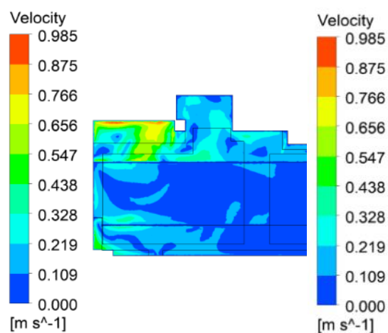
速度云图（改造前）
