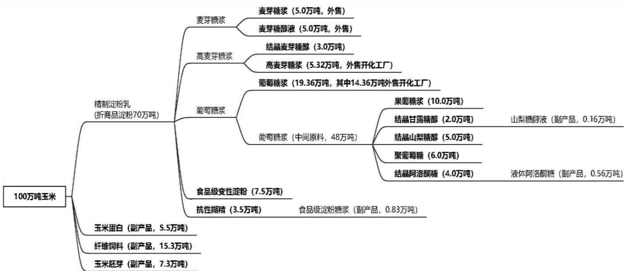
图1 100万吨玉米精深加工健康食品配料项目总工艺流程图
