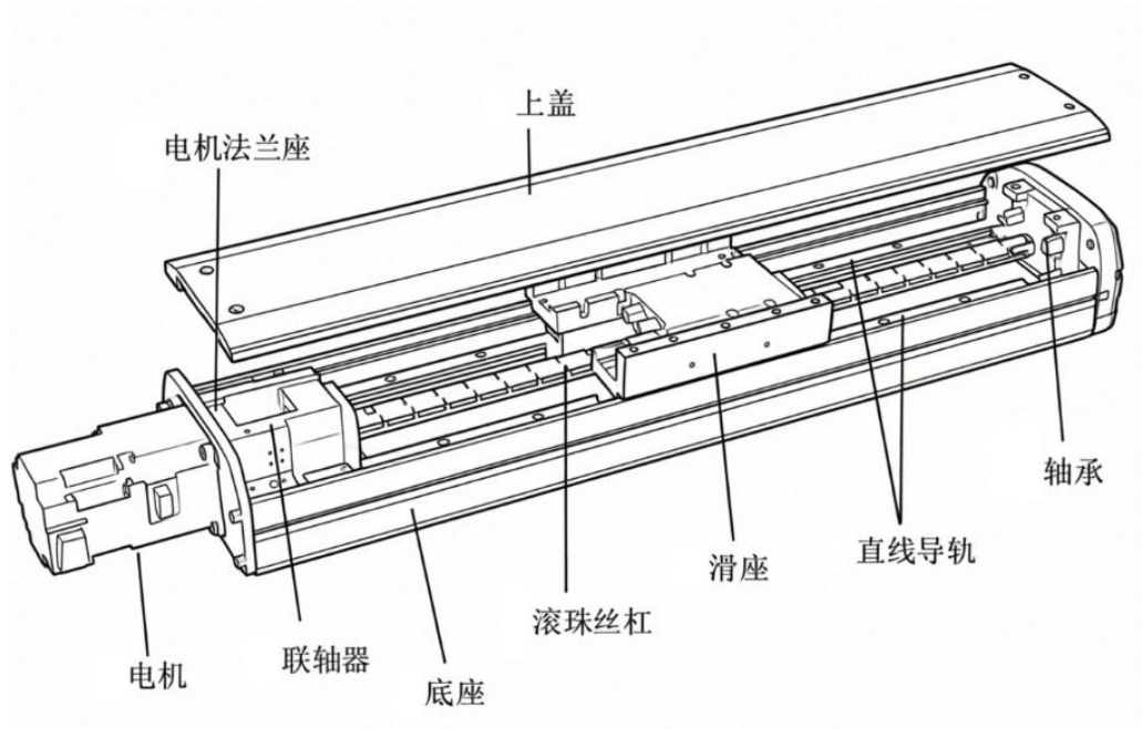
直线传动系统结构示意图
