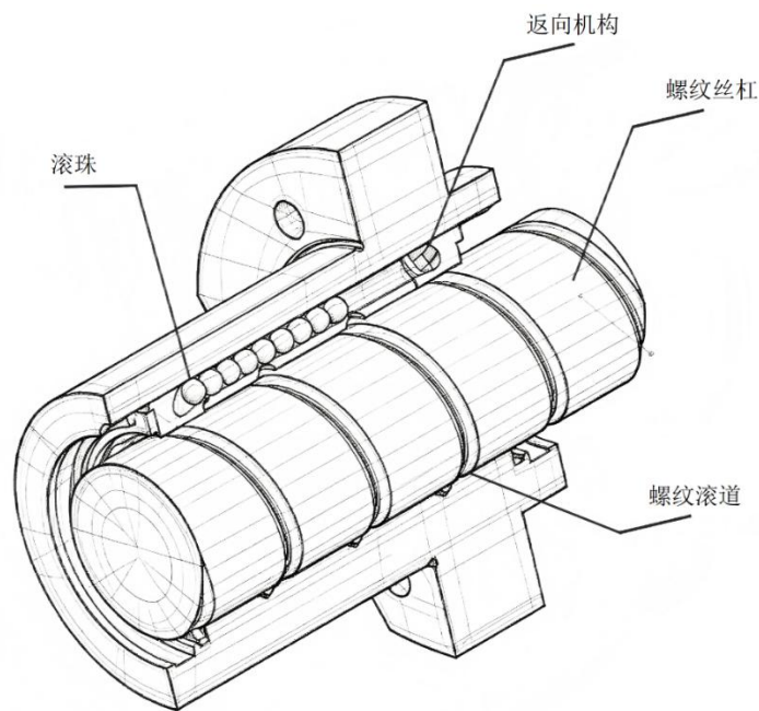
滚珠丝杠副结构示意图
