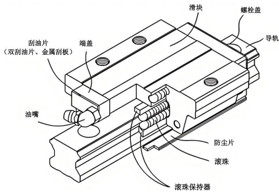
直线导轨副结构示意图
