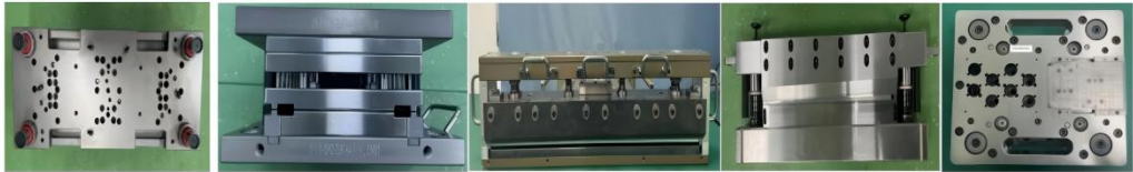
冲压模 负极极耳模具 冲压模具 阵列孔 负极裁切模具 组件陶瓷刀 负极裁切模具 绝缘垫片 冲切模具
