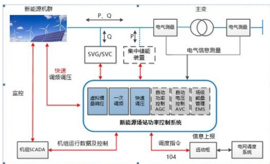
（新能源场站主动支撑功能拓扑图）
