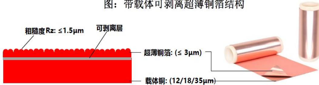
图：带载体可剥离超薄铜箔结构
